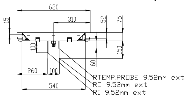
Zij aanzicht
